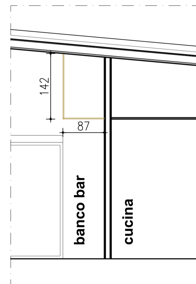
SEZIONE B-B CONTROSOFFITTO IN LASTRA DI CARTONGESSO SOPRA BANCO BAR RETROSTANTE CON MISURE VARIABILI PER PARETE INCLINATA DELLA CUCINA E ATTACCO SU ESISTENTE
