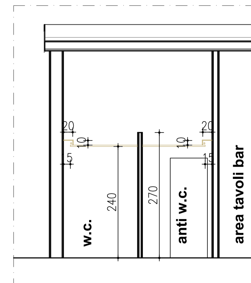
SEZIONE A-A CONTROSOFFITTO IN LASTRA DI CARTONGESSO SOPRA ANTI E W.C., CON NICCHIA NEI W.C. PER INSERIMENTO PUNTO LUCE MENTRE NELL'ANTI SARA' INSERITO FARETTO AD INCASSO
